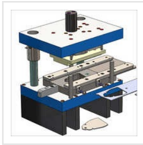
Press Dies Tools
