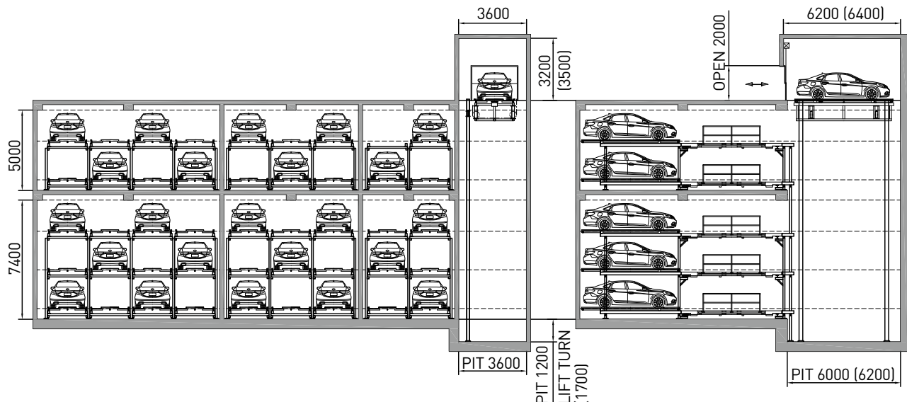
주차장 정면도 Elevation
