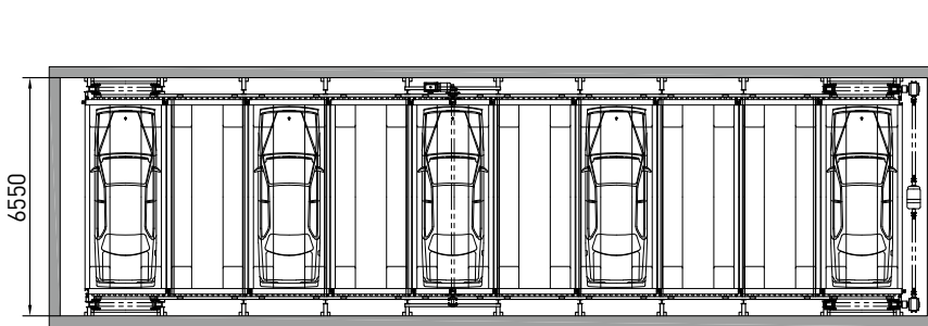
주차장 평면도 Parking Lot Layout
