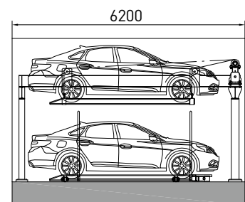
주차장 측면도 Section
