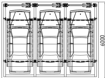
주차장 평면도 Parking Lot Layout
