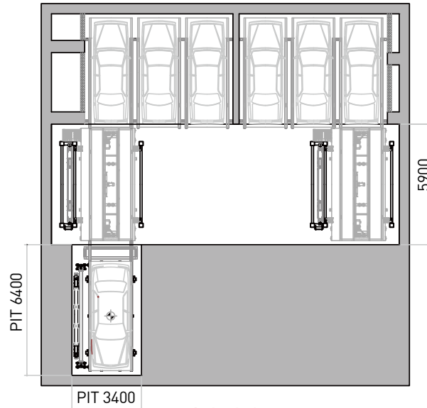
주차장 평면도 Parking Lot Layout
