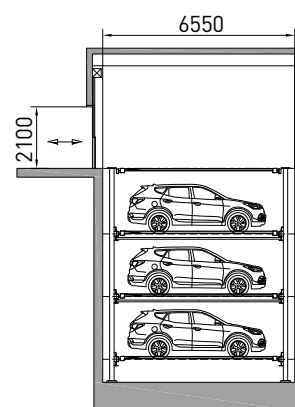
주차장 측면도 Section
