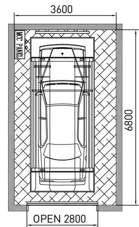
입고층 평면도 Entry Room Layout
