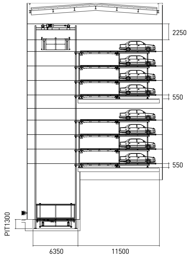
주차장 측면도 Section
