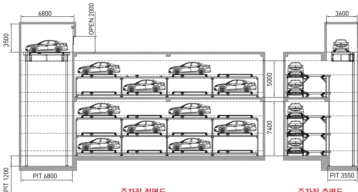
주차장 정면도 Elevation
