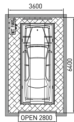
입고층 평면도 Entry Room Layout
