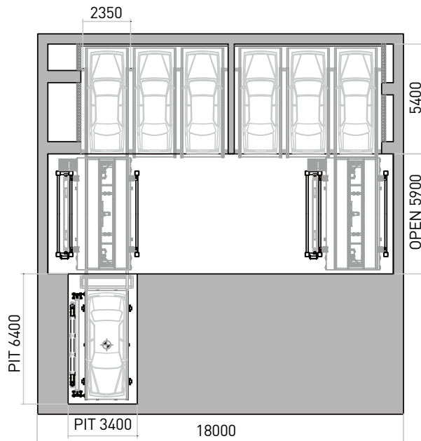
주차장 평면도 Parking Lot Layout
