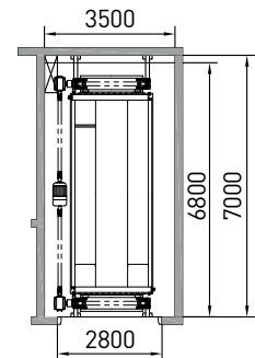
입고층 평면도 Entry Room Layout
