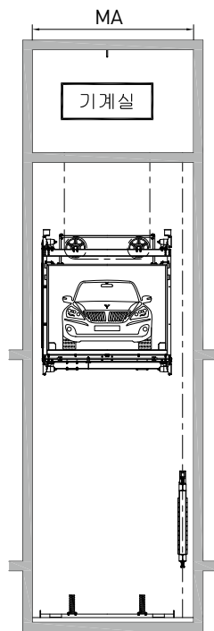
승강로 정면도 Elevation
