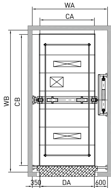
승강로 및 기계실 평면도 Car Lift and Machine Room Layout
