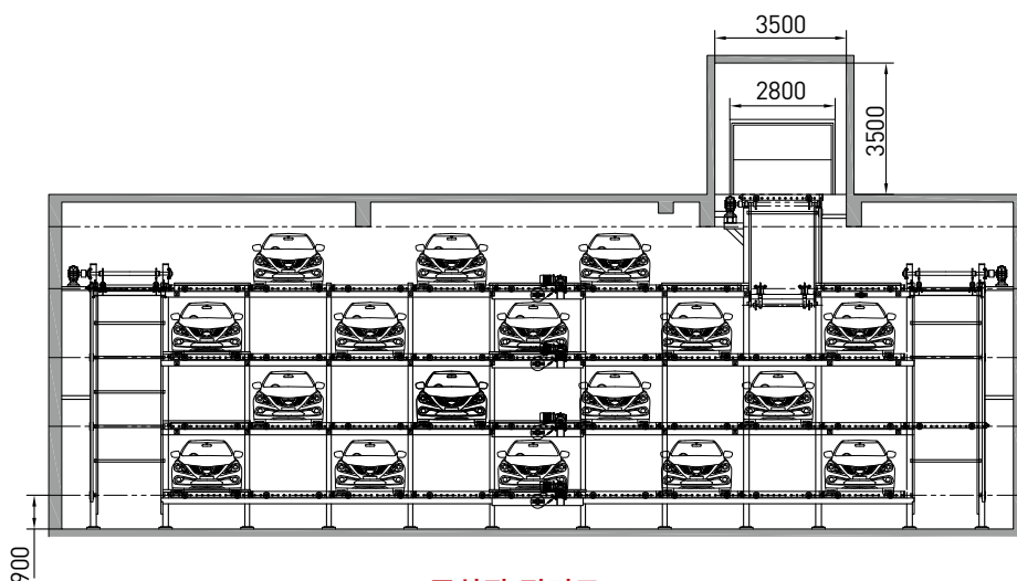
주차장 정면도 Elevation
