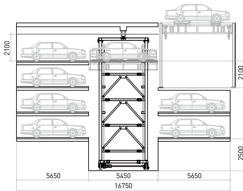
주차장 측면도 Section
