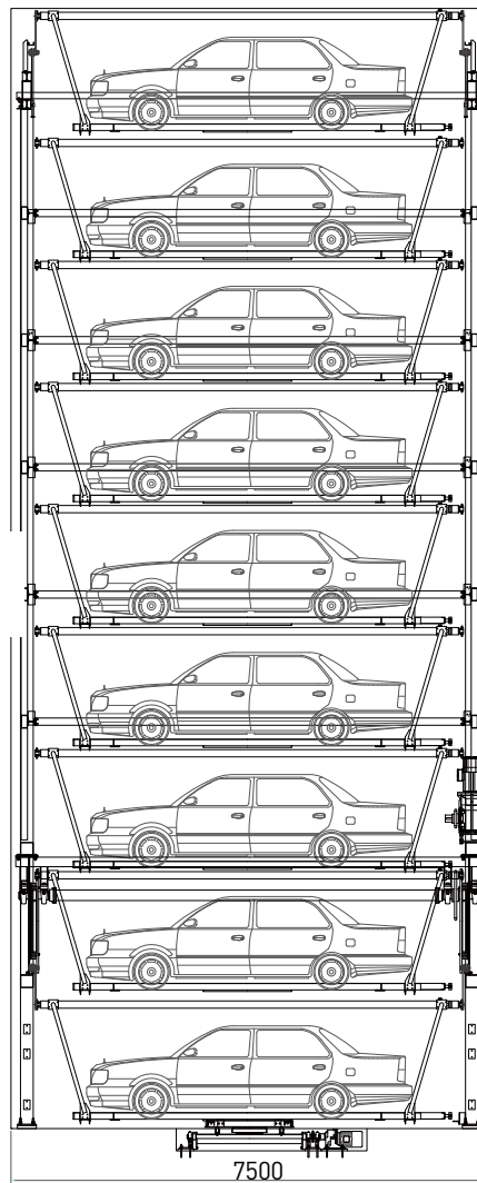
주차장 측면도 Section
