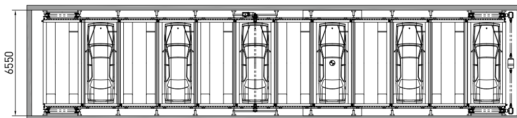
주차장 평면도 Parking Lot Layout
