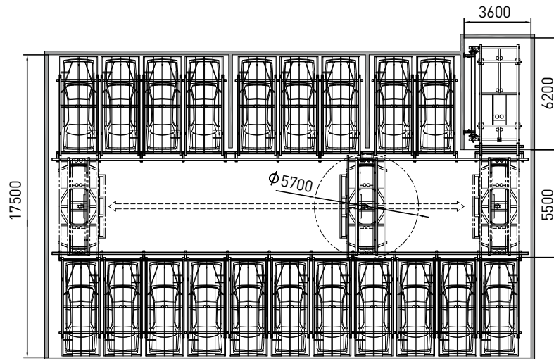
주차장 평면도 Parking Lot Layout
