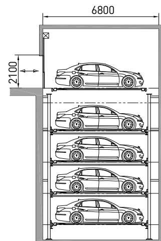
주차장 측면도 Section
