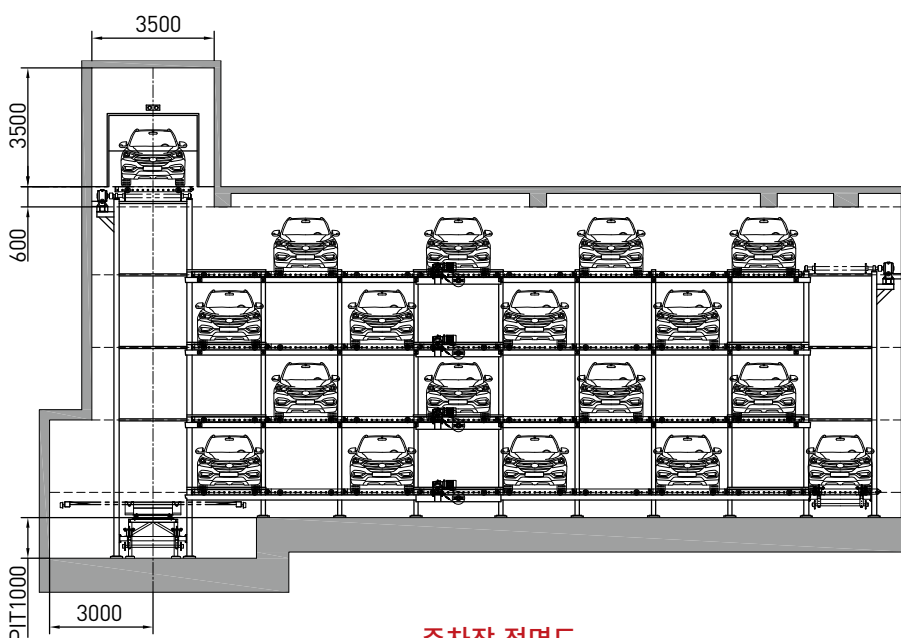
주차장 정면도 Elevation
