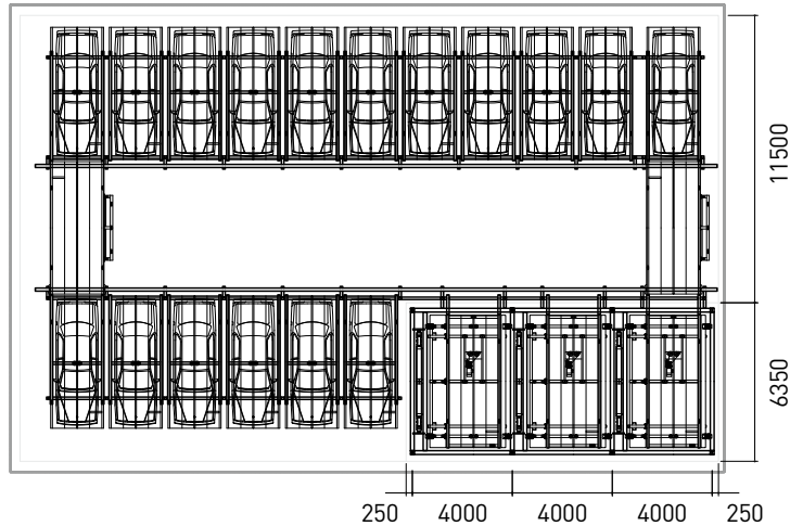
주차장 평면도 Parking Lot Layout
