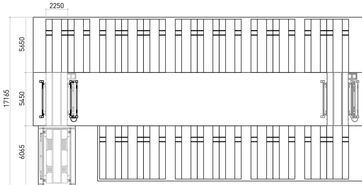
주차장 평면도 Parking Lot Layout
