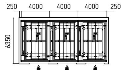
입고층 평면도 Entry Room Layout
