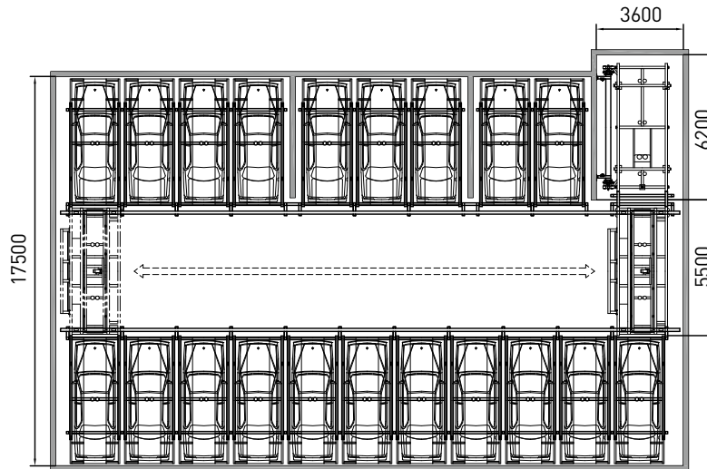
주차장 평면도 Parking Lot Layout
