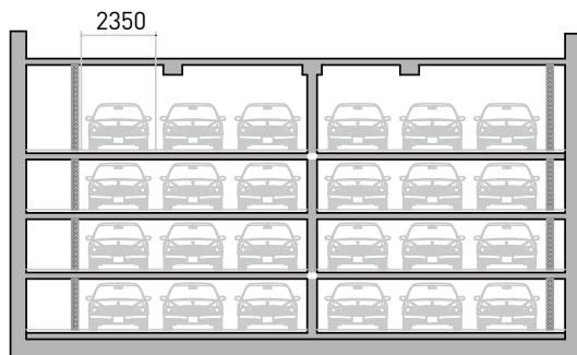
주차장 정면도 Elevation
