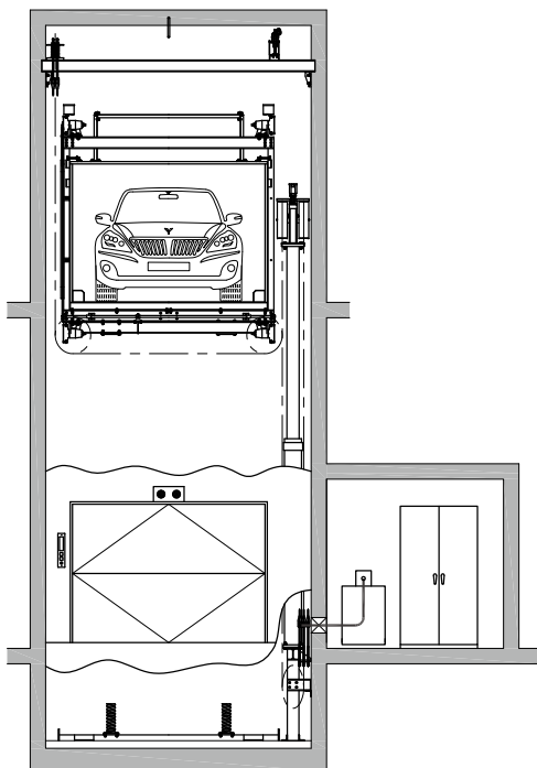
승강로 정면도 Elevation
