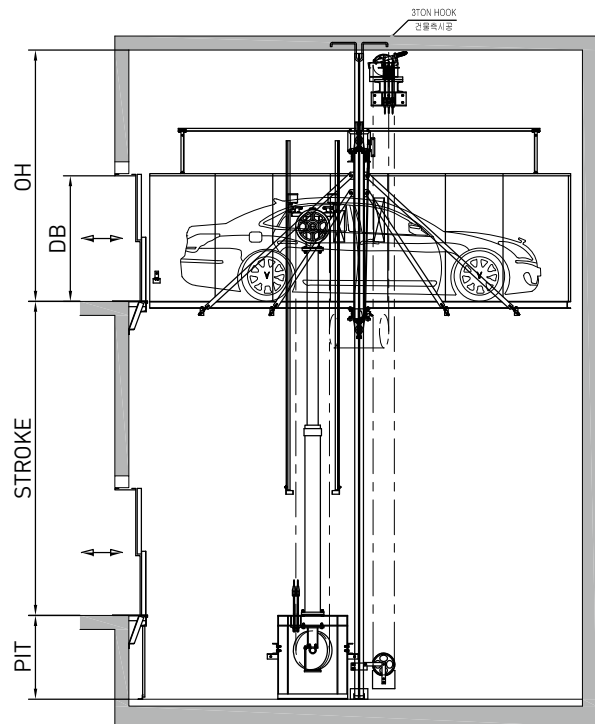
승강로 측면도 Section
