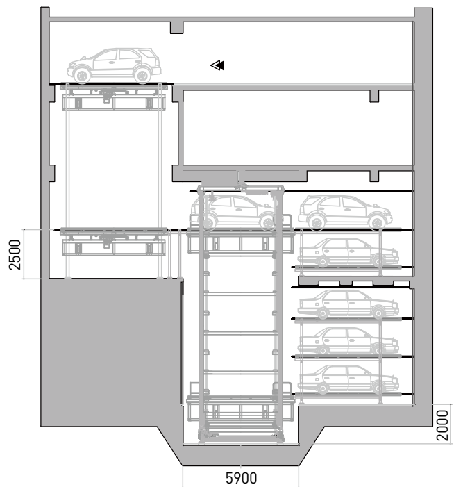
주차장 측면도 Section
