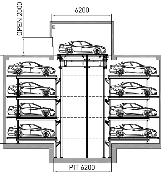
주차장 측면도 Section
