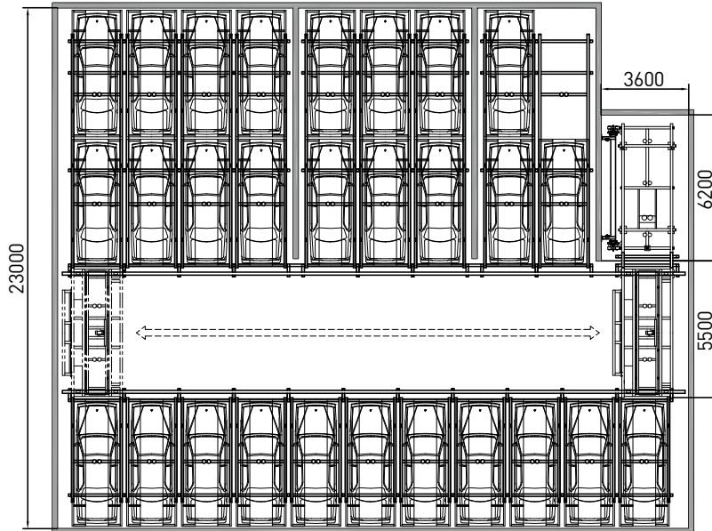
주차장 평면도 Parking Lot Layout
