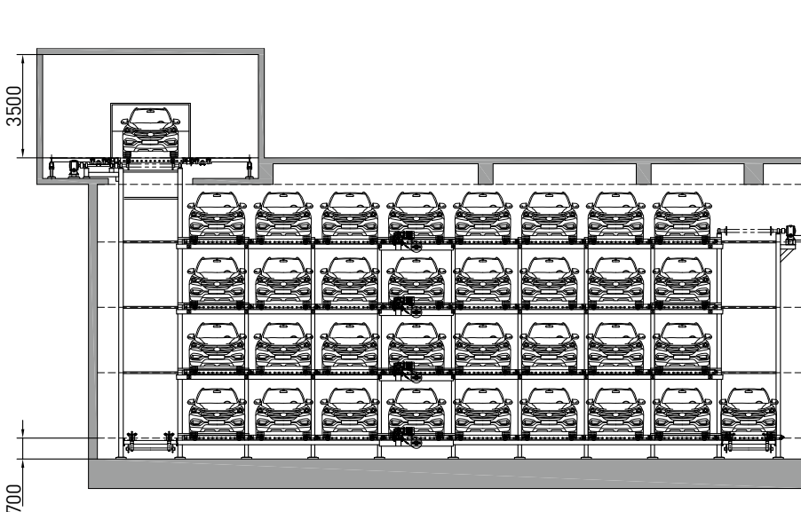
주차장 정면도 Elevation
