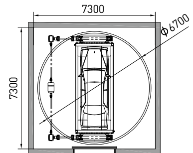
입고층 평면도 Entry Room Layout
