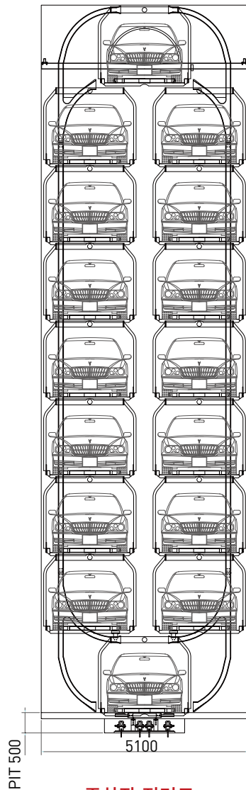
주차장 정면도 Elevation
