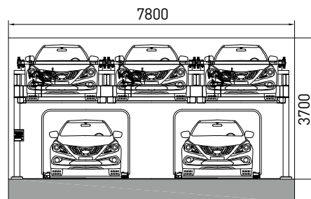
주차장 정면도 Elevation
