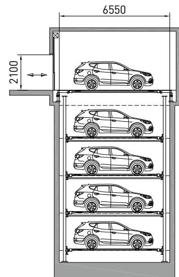
주차장 측면도 Section
