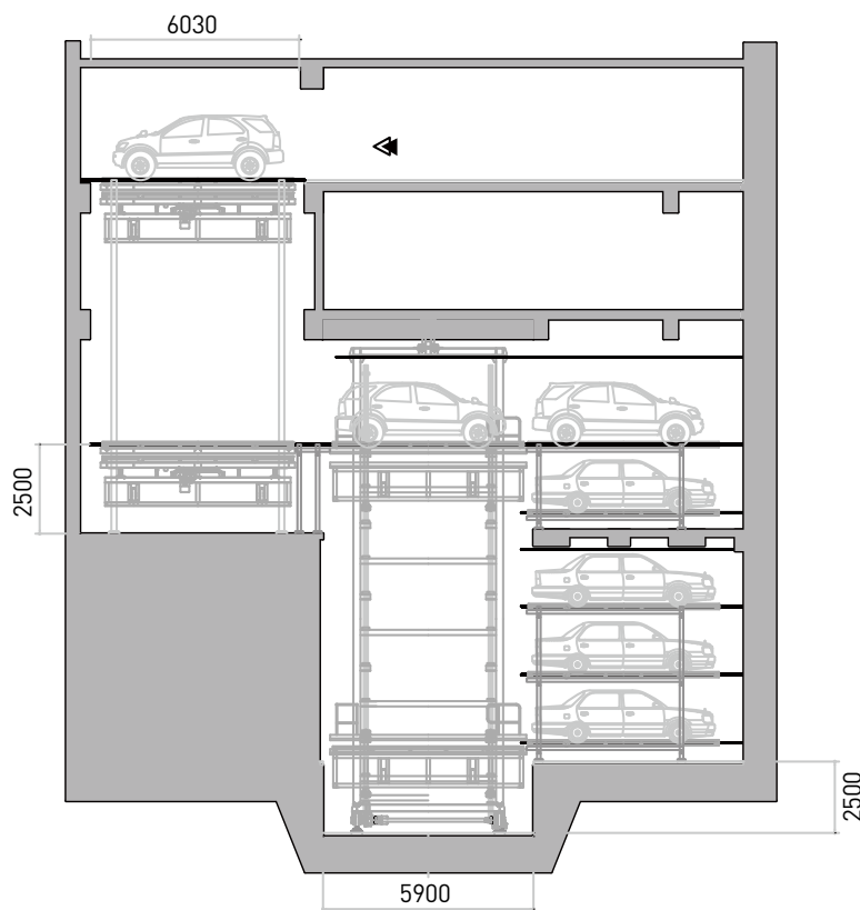
주차장 측면도 Section
