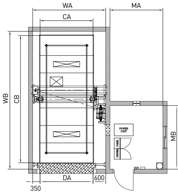
승강로 및 기계실 평면도 Car Lift and Machine Room Layout
