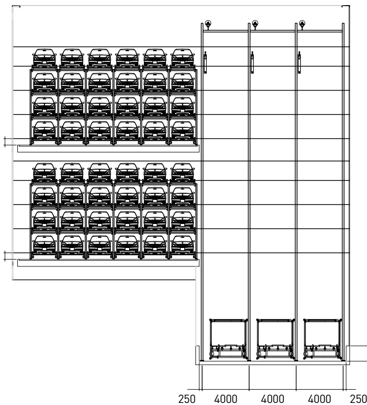
주차장 정면도 Elevation
