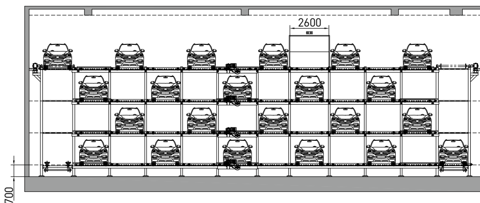
주차장 정면도 Elevation
