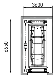
입고층 평면도 Entry Room Layout
