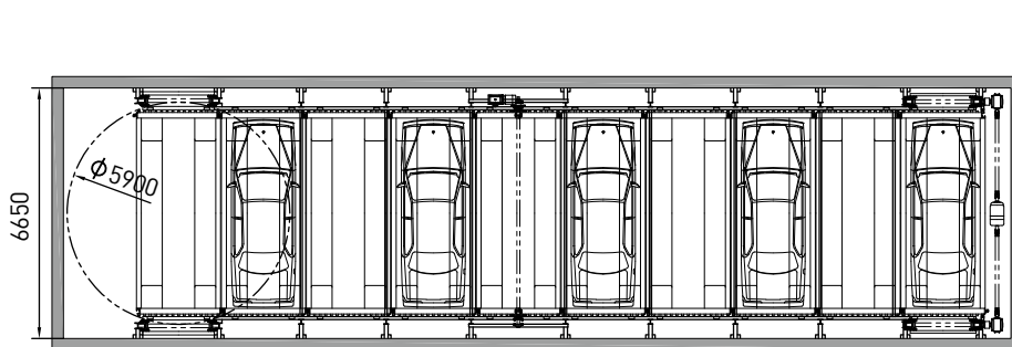
주차장 평면도 Parking Lot Layout
