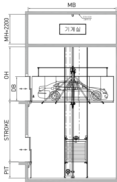
승강로 측면도 Section
