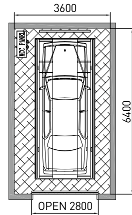
입고층 평면도 Entry Room Layout
