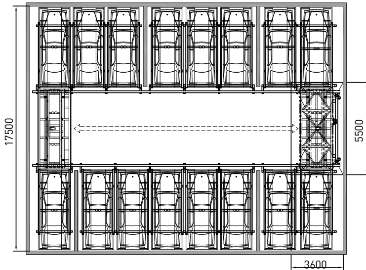
주차장 평면도 Parking Lot Layout
