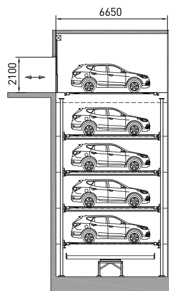
주차장 측면도 Section
