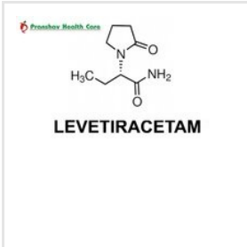
Levetiracetam IP
