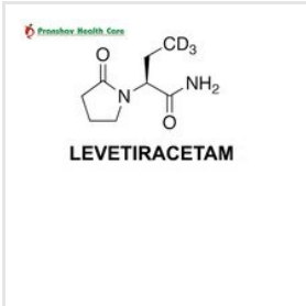
Levetiracetam
