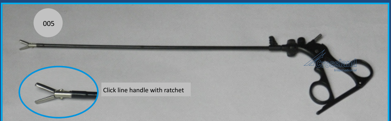
005 : CL-LAP-005 : Non-teeth Grasping forceps.
