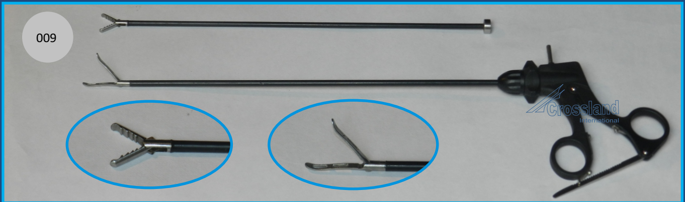
009 : Grasper forceps : (I) : Crocodile forceps - CL-L / INS / 008-09., (J) : Bowel Grasper forceps - CL-L / INS / 10.
