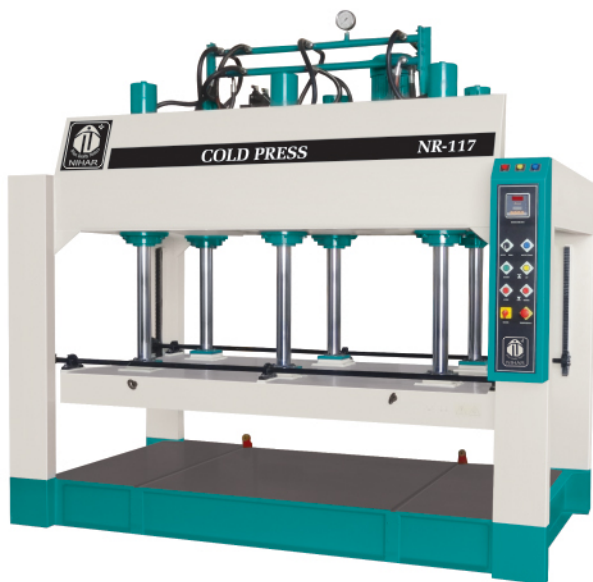
Cold Press (150 Ton)
