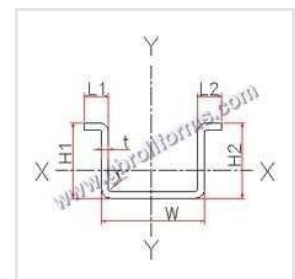
Top Hat Section
