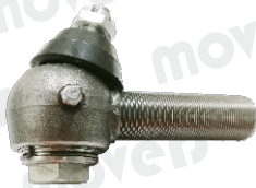
1009 1009A 30X1.5 RH DRAG LINK END TATA 2416 RH TURBO 28X1.5, 27 NO. NUT
