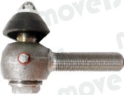
1079 TIE ROD END 2515 EX R&L 24X1.5mm, THICK GOLI 27 No. NUT
