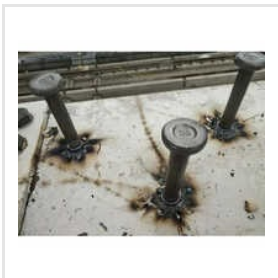
Shear Connector Stud
