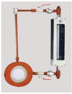
Rotameter -Bye Pass
