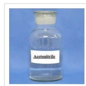
Acetonitrile
