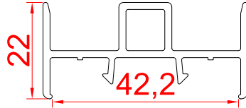
Sliding Sash Connector RSA - 22 SA
