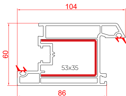
Casement Inward Door Sash RSC - 104 ID
