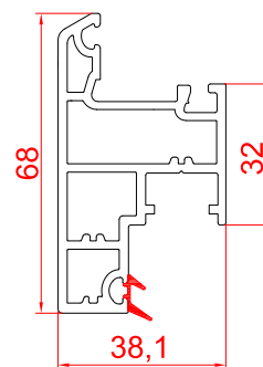
Openable Mesh RSM - 68 OM
