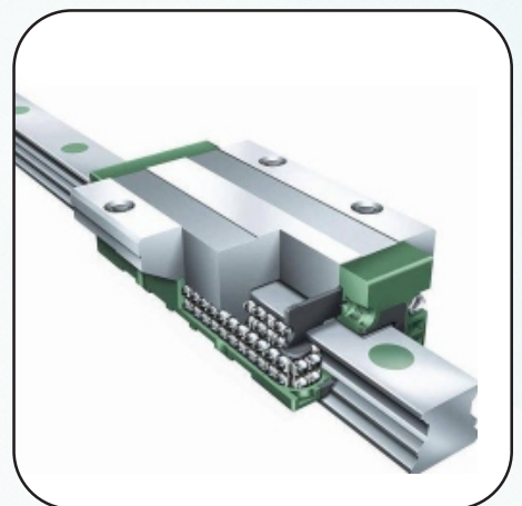
200mm Linear Guide
