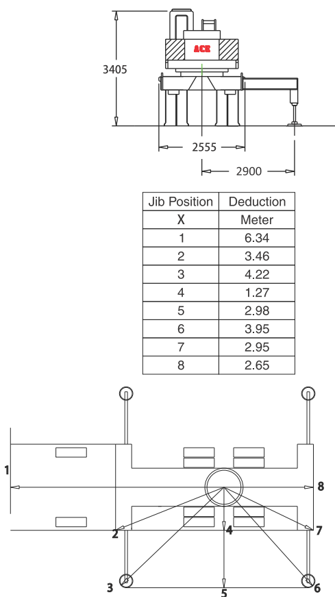
Dimensions
