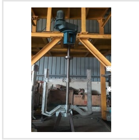
Anchor Type Agitator
