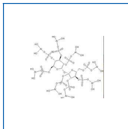
SUCRALFATE USP
