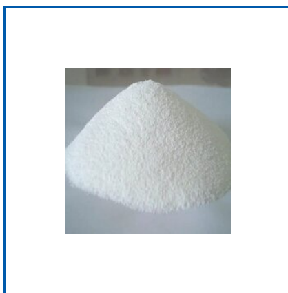
CARBAMAZEPINE IP/BP/USP
