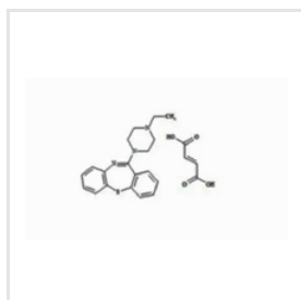
Quetiapine Fumarate
