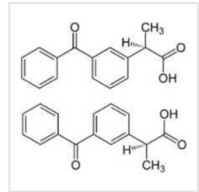
KETOPROFEN IP/BP/USP
