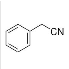
Benzyl Cynaide
