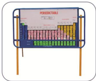
Periodic Table
