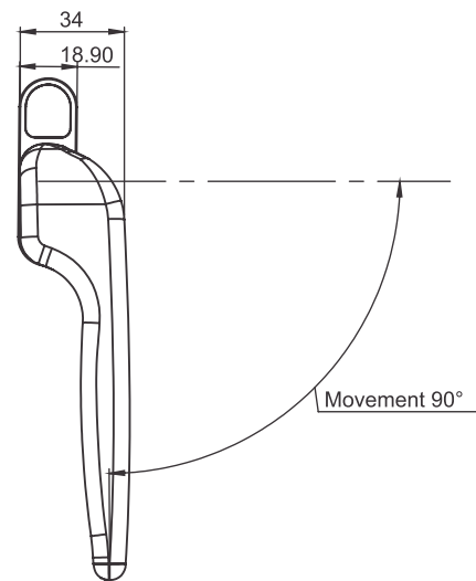
Espagnolette Offset Handle Code PL10125L/25R
