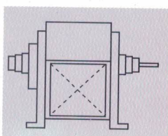
No 3 - SWSI No 3 - DWDI
