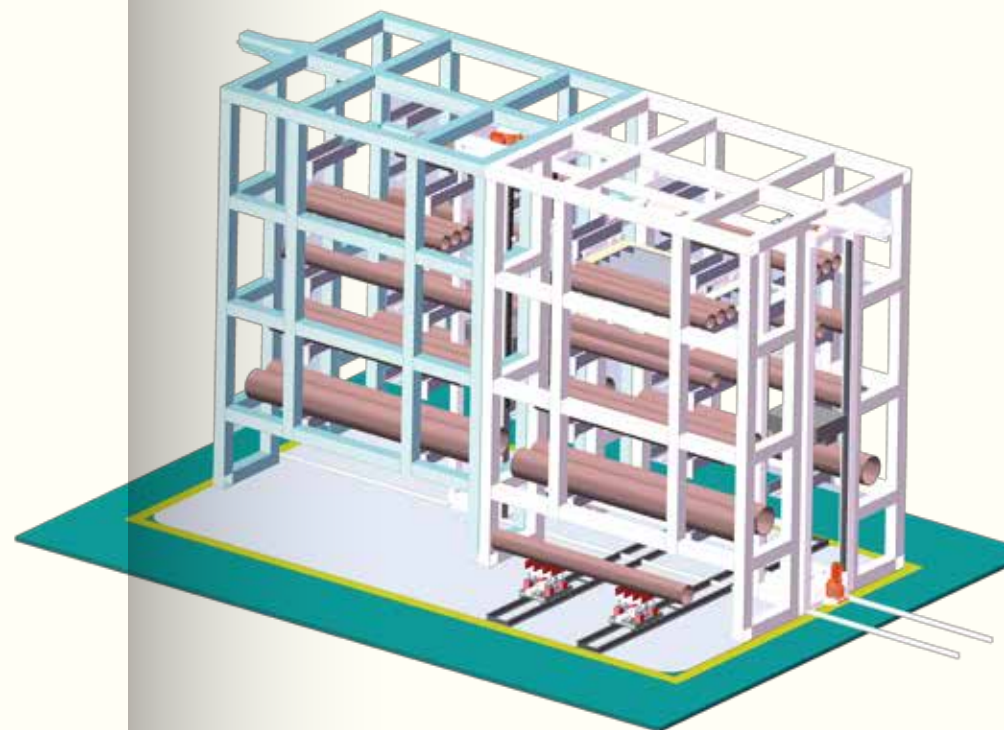
立体仓库效果图1
