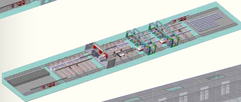
移动车间式管道预制解决方案
