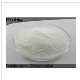
Sodium Benzoate
