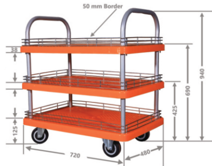
PT-150/300/500-3LB
