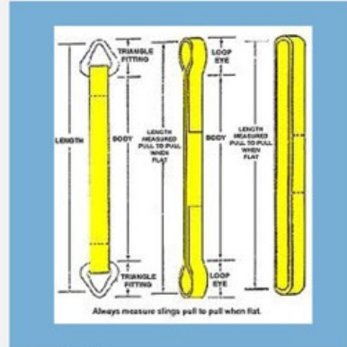
Web Sling
