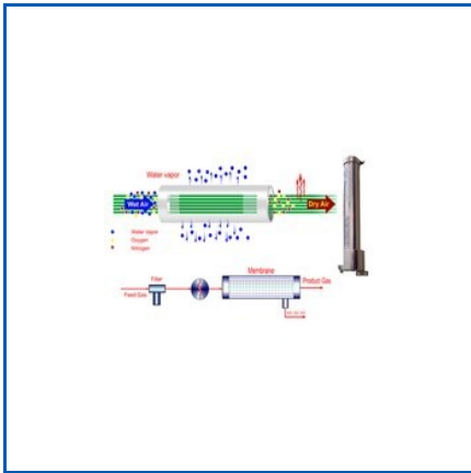
MEMBRANE DRYER
