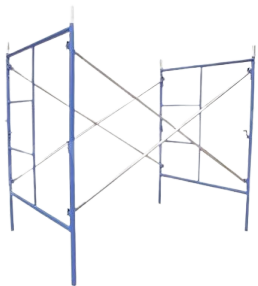
H-Frame
