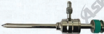
ASW 57 | TROCAR & CANNULA 7 MM
