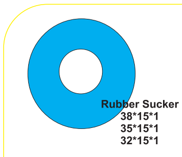
Rubber Sucker 38*15*1 35*15*1 32*15*1
