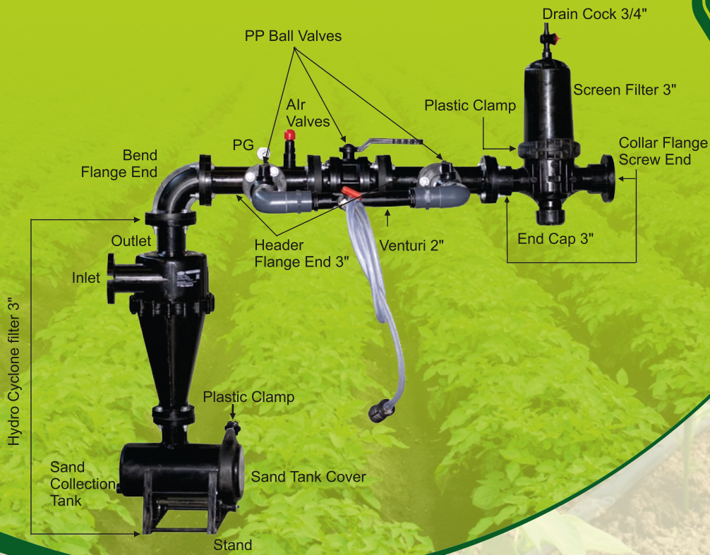
HydroCyclone (2", 2.5", 3")
