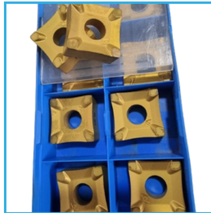
OD SCARFING INSERTS
