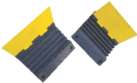
Code : JS 009 Rubber Cable Protector Size : 500 x 470 x 50 mm
