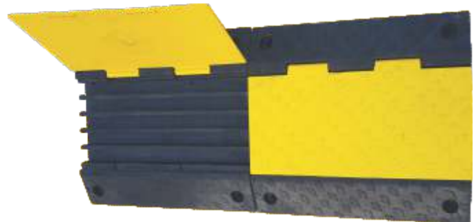
Code : JS 009 Rubber Cable Protector Size : 500 x 470 x 50 mm
