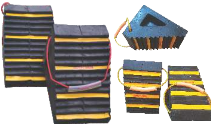
Code : JS 025 Rubber Wheel Chock Size : 250 x 170 x 182 mm
