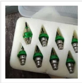
Juki Nozzles
