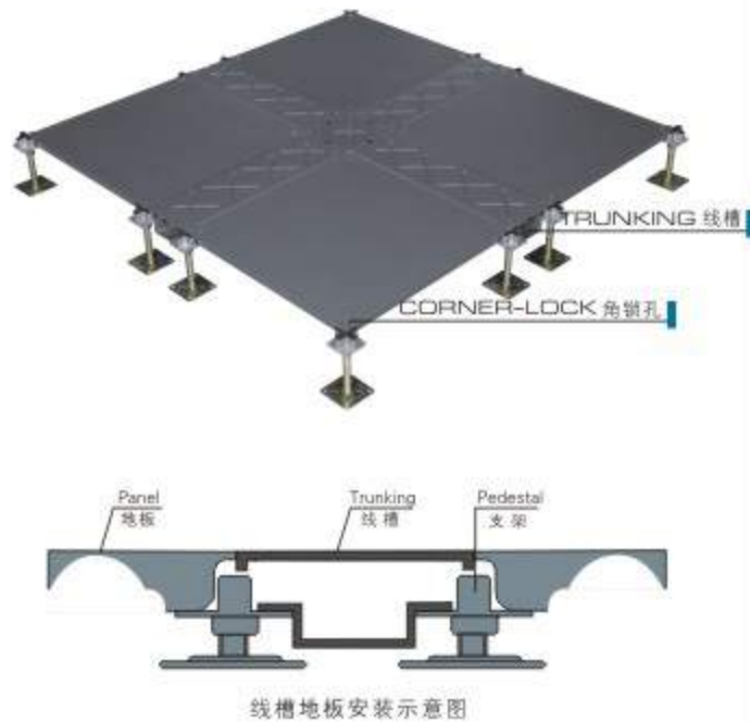
线槽地板安装示意图
