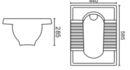
ORISA PAN 23 Pan 585 x 440 x 285 MM
