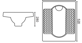
ORISA AQUA 20 Pan 520 x 430 x 280 MM
